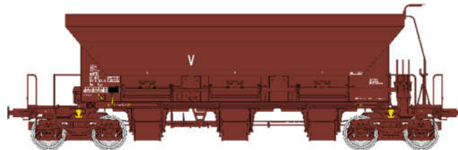
Réf. WB-804 : WAGON TREMIE A BALLAST F70 Uas « INFRA V » SNCF Ep. VI
