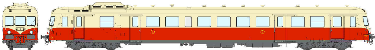
Autorail X 2828 version d'origine, Rouge 605 et Crème 407, LYON-VAISE, SNCF Ep. III.
